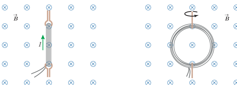
شکل ۳-۲۶ با چرخاندن پیچه درون میدان مغناطیسی \vec{B} ، زاویه بین میدان مغناطیسی و سطح پیچه تغییر می‌کند. این تغییر زاویه سبب القای جریان در پیچه می‌شود.
