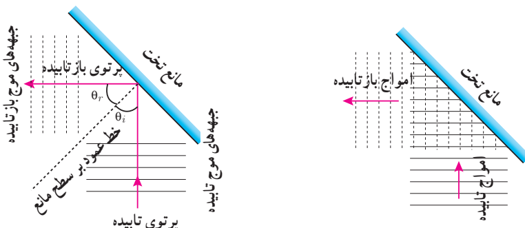
شکل ۳-۳۲ طرحی از جبهه‌های موج تابیده (خطوط توبر) و جبهه‌های موج بازتابیده (خطوط خطین) شکل ۳-۳۳ نمودار پرتویی همراه با جبهه‌های موج برای بازتاب امواج تخت از سطح مانعی تخت
