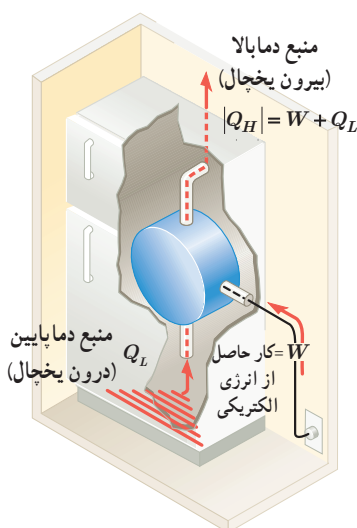
شکل ۸-۵ طرز کار طرح وار یک یخچال خانگی
