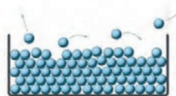
شکل ۴-۲۳ در حین تبخیر سطحی، مولکول‌های پراورزی‌تر از سطح مایع می‌گریزند.
