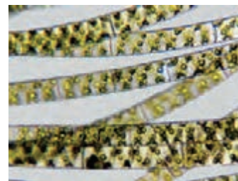
شکل ۷. پریاخته‌ای ساده
