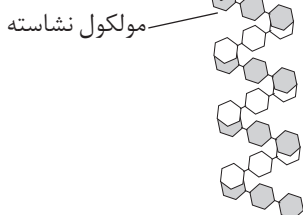
شکل ۱۹- الگوی تبدیل نشاسته به مونومرهای سازنده آن
