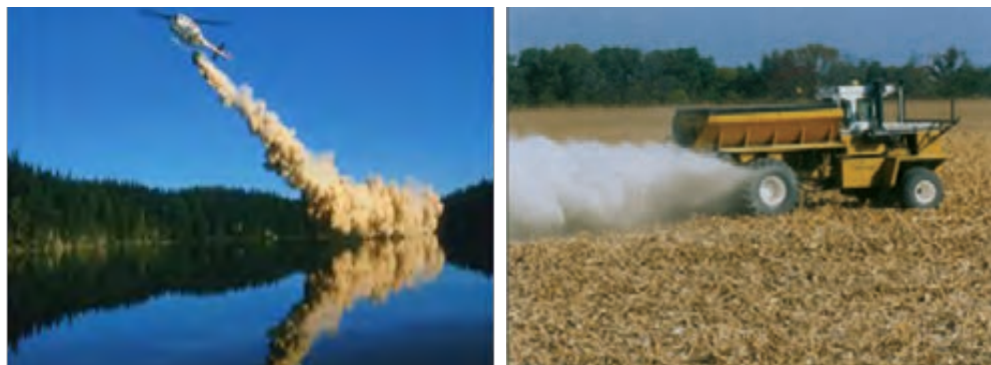
شکل ۱۴- افزودن آهک به زمین‌های کشاورزی و دریاچه‌های اسیدی
