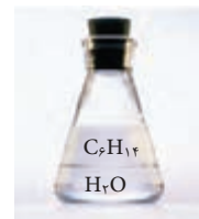
(الف) آب و هگزان
