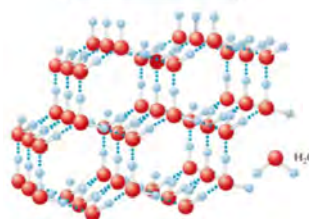
شکل ۱۹- حلقه‌های شش‌ضلعی مبنای شکل دانه‌های برف.
