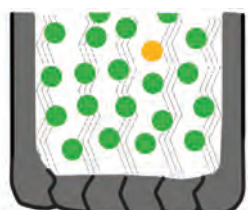
شکل ۲۴- سوختن گاز هیدروژن
