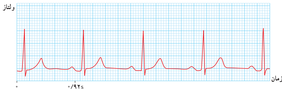
شکل ۱-۳ ب نمونه‌ای از نمودار الکتروقلب نگاره ۱ (نوار قلب) یک شخص
