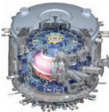
شکل ۱۵-۶ طرحی از راکتور آزمایشی گرما هسته‌ای بین‌المللی (ITER) ۱ . ساخت این راکتور با مشارکت چندین کشور جهان، از سال ۲۰۰۷ در فرانسه شروع شده است و قرار است از سال ۲۰۳۵ با توان خروجی ۵۰۰ مگاوات شروع به کار کند.
