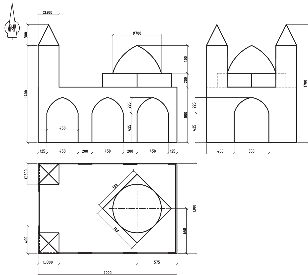
شکل ۹-۱۲. نقشه نمای مسجد
