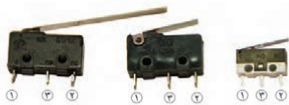
ب) چند نمونه میکروسوییچ
