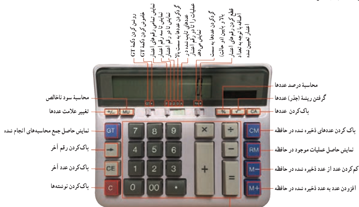
شکل ۱۰-۸. کاربرد دکمه‌های ماشین حساب رومیزی
