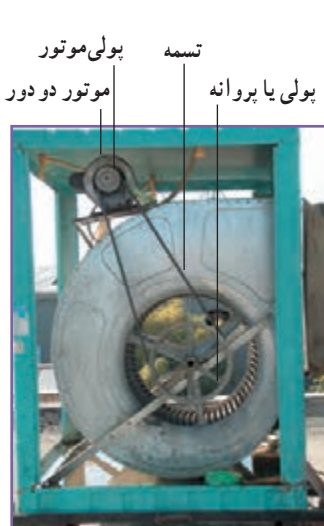
ب۔ نمای سمت پولی پروانہ کولر آبی
