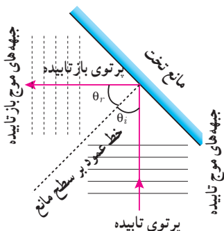
شکل ۴-۶ طرحی از جبهه‌های موج تابیده (خطوط توپر) و جبهه‌های موج بازتابیده (خطوط خط‌چین) شکل ۴-۷ نمودار پرتویی همراه با جبهه‌های موج برای بازتاب امواج تخت از سطح مانعی تخت
