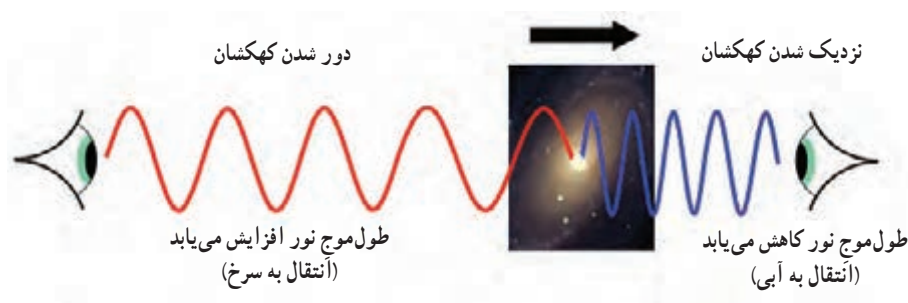
شکل ۲۹-۳ اگر کهکشانی به ما نزدیک یا از ما دور شود، بسامد و طول موج دریافتی از آن تغییر می‌کند.
