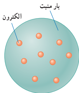
شکل ۵-۹ در مدل تامسون، بار الکتریکی مثبت به طور همگن در کره‌ای توزیع شده است و الکترون‌ها مانند کشمش‌های کیک در نقاط مختلف آن قرار دارند.
