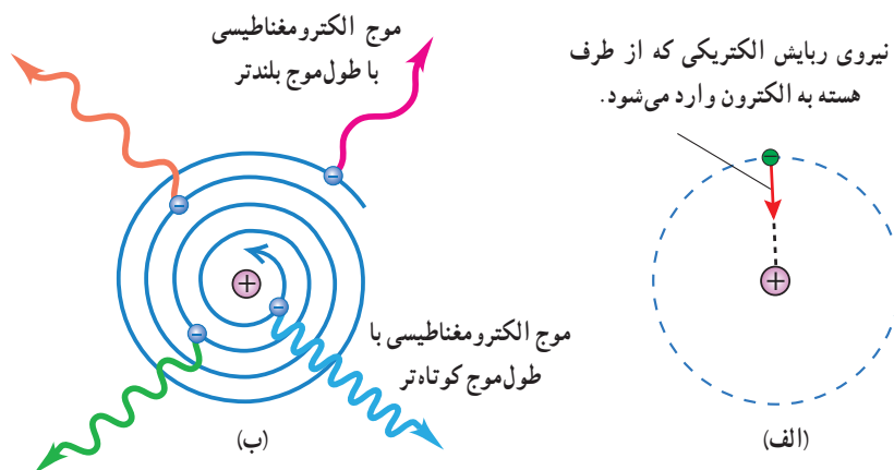
شکل ۴-۹ ناتوانی مدل اتم رادرفورد در تبیین پایداری اتم. الف) اگر الکترون
