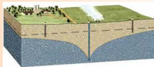
شکل ۲. چاه بهره‌برداری
