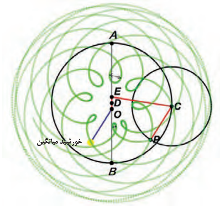
مجموعهٔ حرکات بازگشتی مریخ، رصدها نشان می‌دهند که مقدار بازگشت مریخ در نزدیکی نقطهٔ اوج A بزرگ‌تر از مقدار بازگشت در نزدیکی نقطهٔ حضیض B است. بطلمیوس برای توضیح این مشاهده نقطهٔ معدل المسیر را فرض می‌کند تا سرعت فلک حامل را تنظیم کند.
