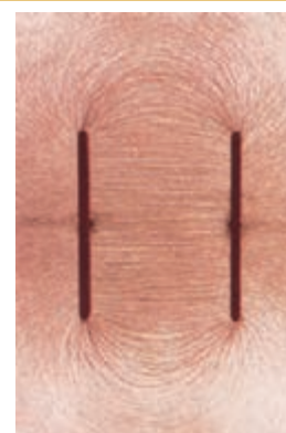
شکل ۱۹-۱ سمت‌گیری دانه‌ها در فضای بین دو الکتروود صفحه‌ای موازی
