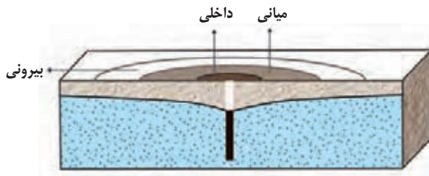
شکل ۵-۳- پهنه‌های حفاظتی چاه آب
