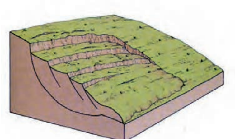
ب) لغزش
