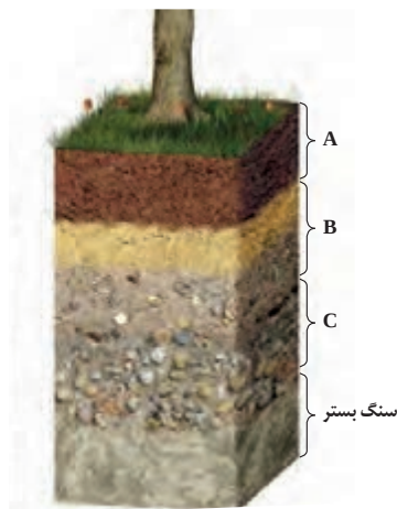
شکل ۸-۳- افق‌های خاک و سنگ بستر
