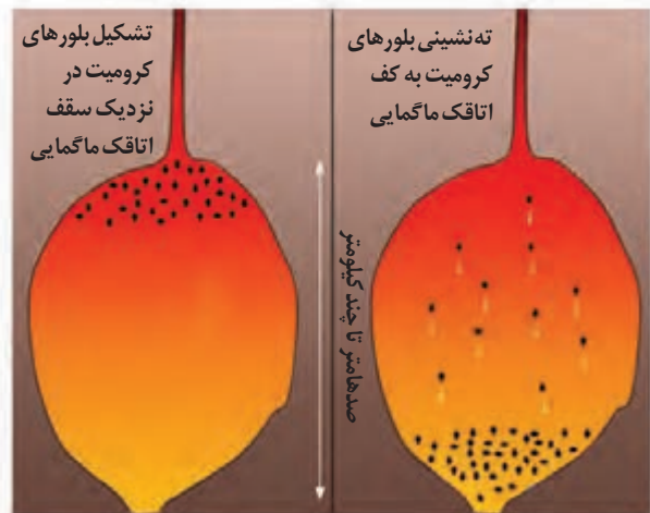
شکل ۴-۲. چگونگی تشکیل و ته نشینی بلورهای کرومیت در اتاقک ماگمایی
