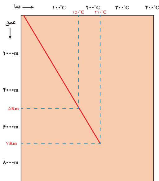
شکل ۶-۲. نمودار شیب زمین گرمایی
