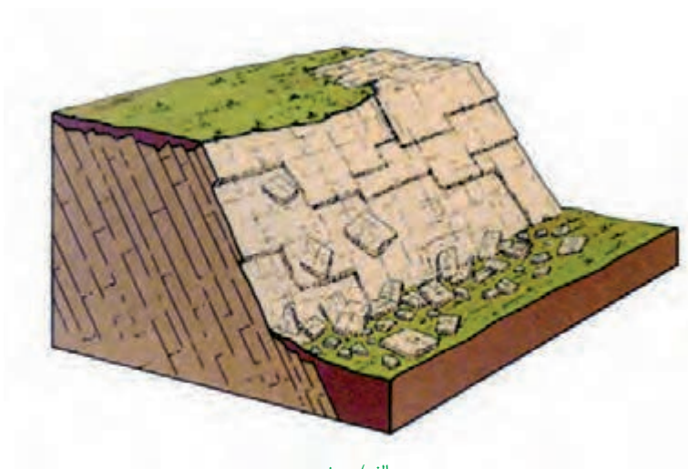
الف) ریزش
